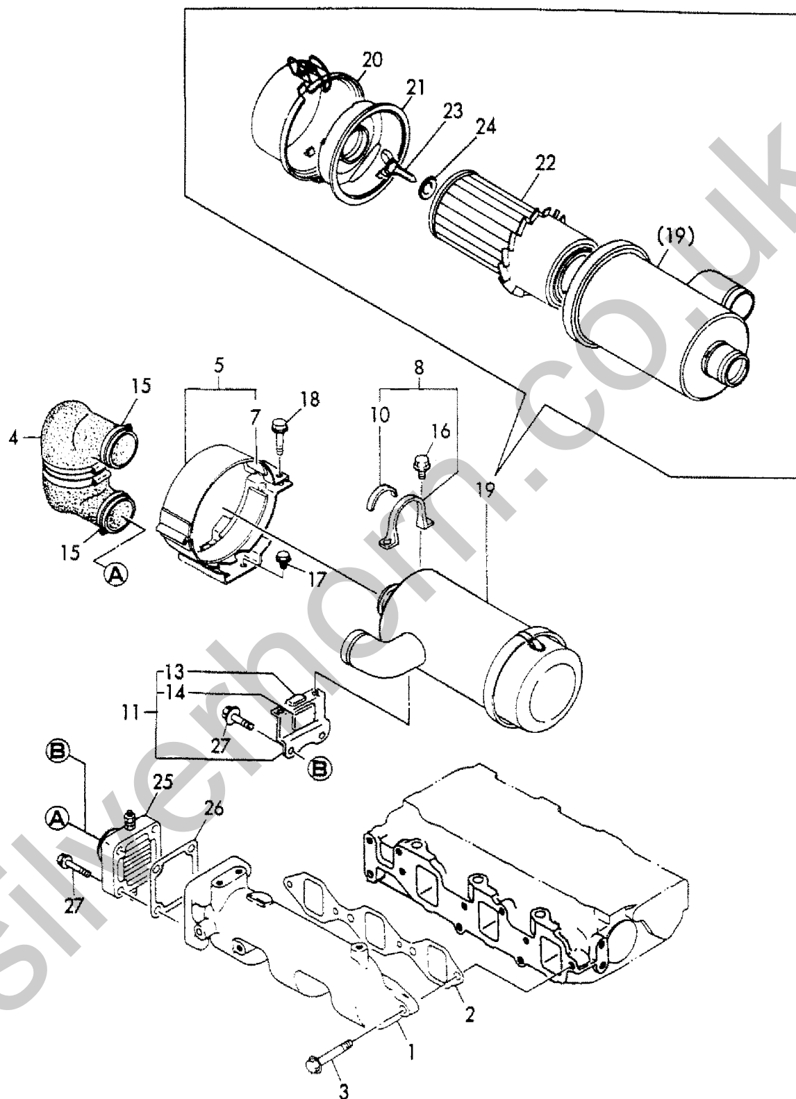
Fig. 5 吸気マニホールド&エアクリーナ SUC. MANIFOLD & AIR CLEANER
