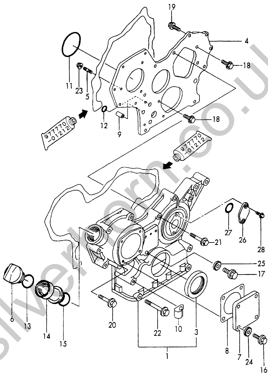
Fig. 2 ギヤケース GEAR HOUSING
